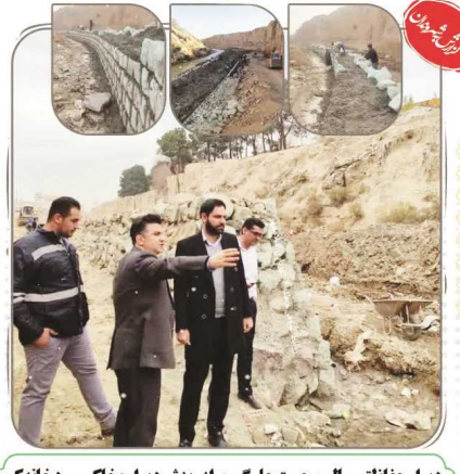
دیوار حفاظتی مالون جهت جلوگیری از ریزش دیوارهای رودخانه کن به طول ۱۰۰ متر به صورت پلکانی با ارتفاع هر پلکان ۴ متر
