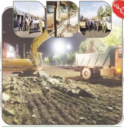
پروژه عملیات عمرانی خیابان ۲۴ مجتمع صنفی خدماتی اسلامشهر شامل زیرسازی، هدایت آب‌های سطحی (جدول گذاری) و روکش مکانیزه آسفالت به مساحت ۲۴۰۰ مترمربع
